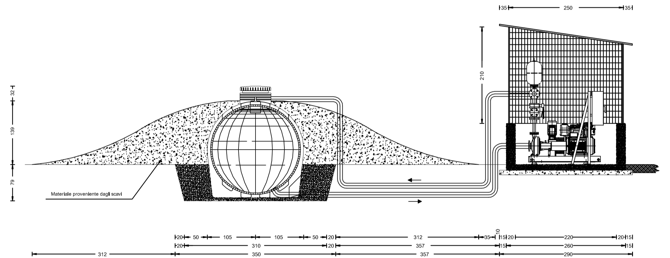
SEZIONE G - H rapp. 1:50
